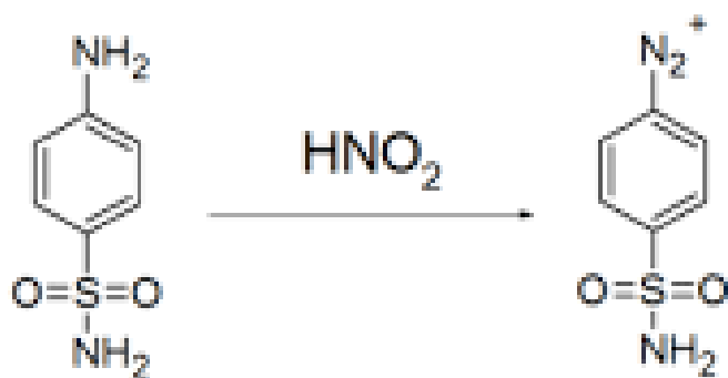
szulfanilamid
