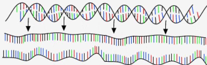
Step 1 : denaturation
