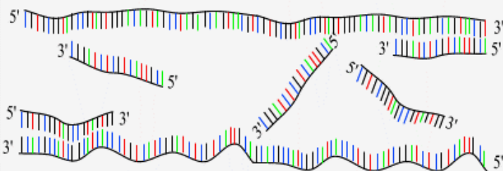
Step 2 : annealing
