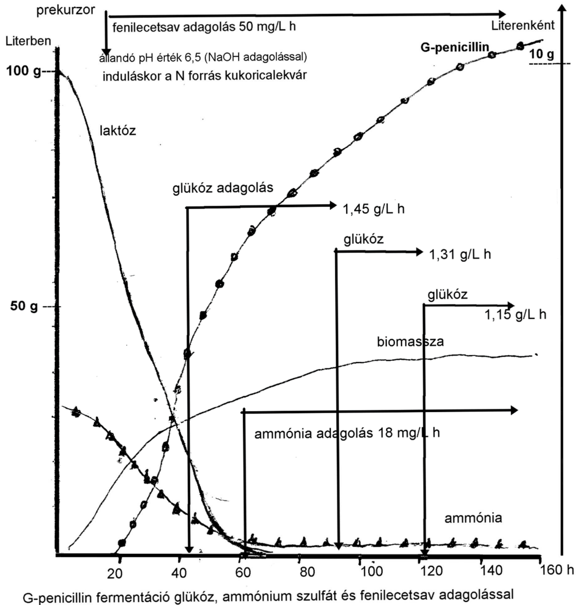
11. ábra Penicillin fermentáció lefutása
