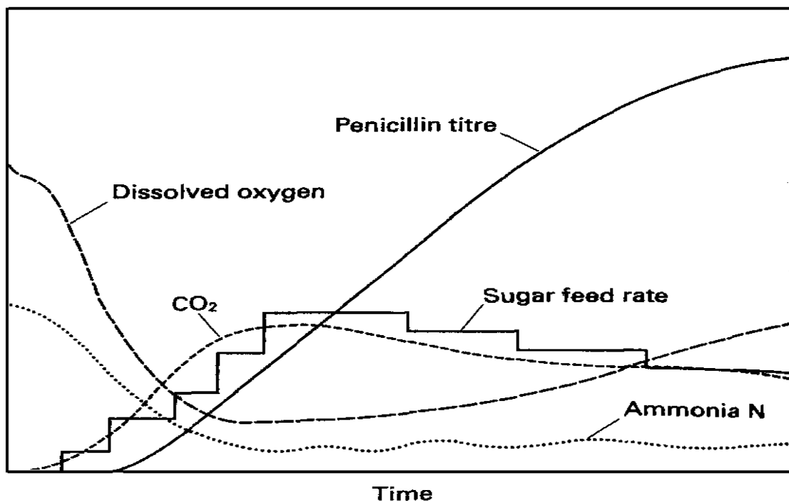
12. ábra: Koncentrációk alakulása a penicillin fermentáció során
