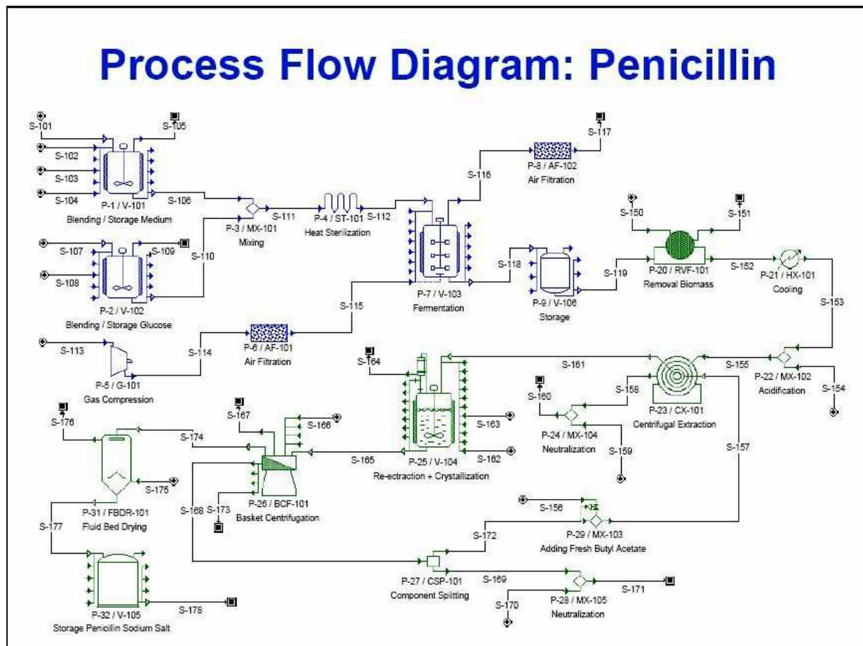
13. ábra A penicillin gyártás folyamatábrája
