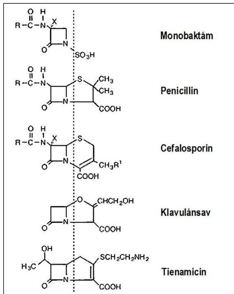
21. ábra Béta-laktám vázas metabolitok
