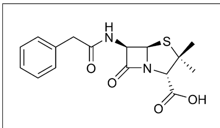
4. ábra A G-penicillin szerkezete
