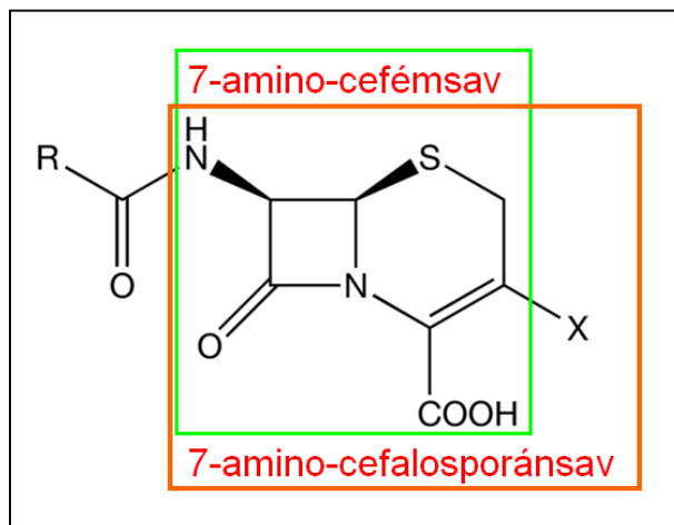
19. ábra A cefalosporin molekula szerkezete
