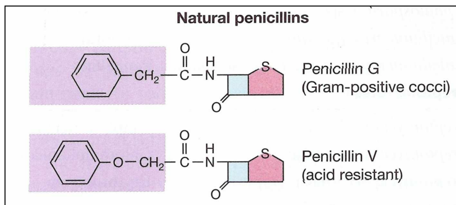
17. ábra Fermentációval előállított penicillinek
