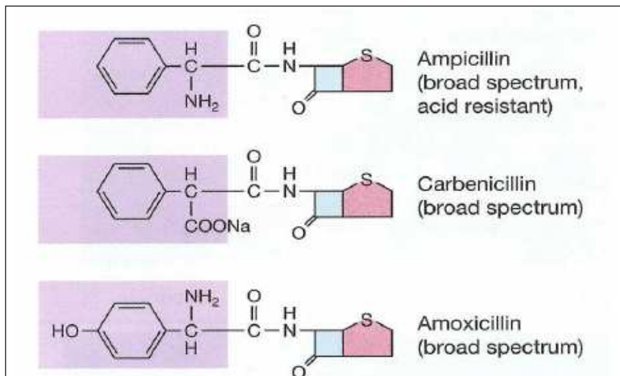
18. ábra: Félszintetikus penicillinek
