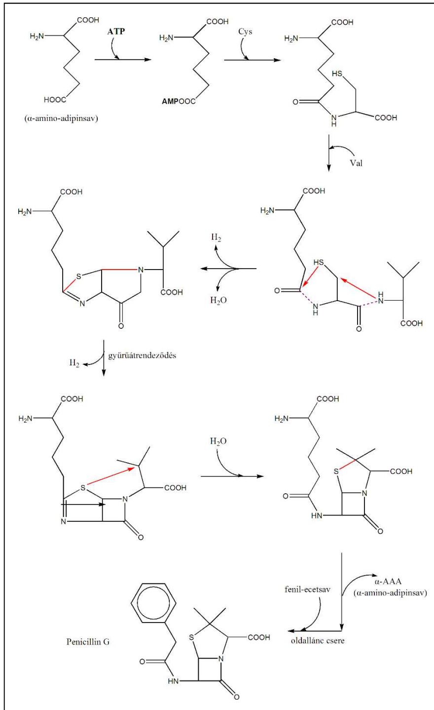
8. ábra A penicillin G bioszintézisének fő lépései
