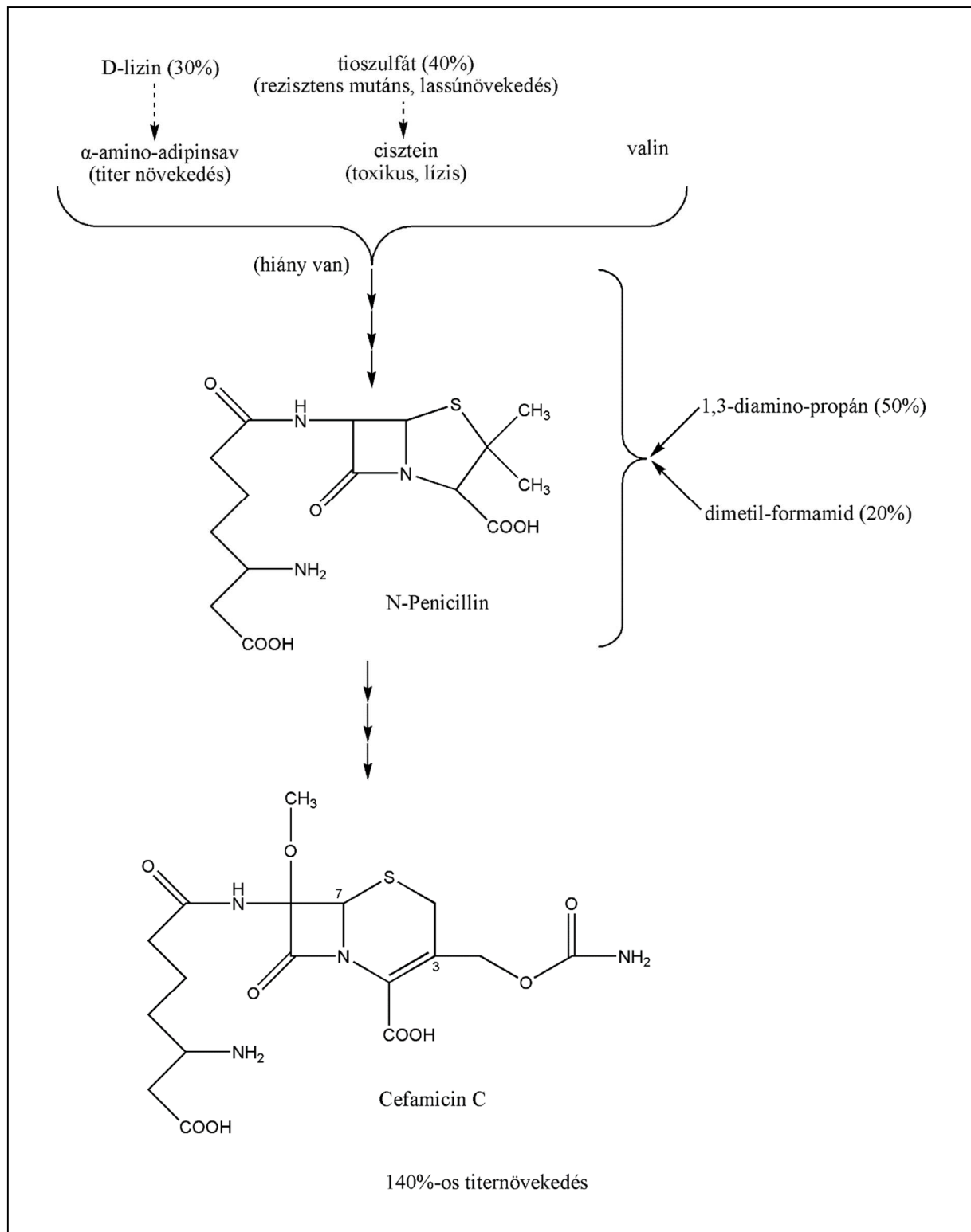
20. ábra Cefalosporin prekurzorok
