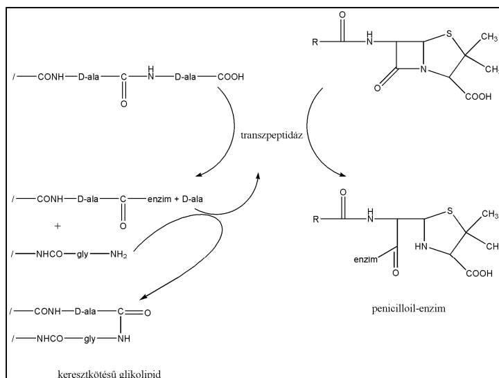
16. ábra A penicillin bekötődése a transzpeptidáz kötőhelyére
