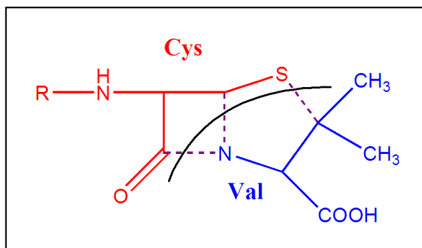
5. ábra A 6-APA alapváz két aminosavból tevődik össze
